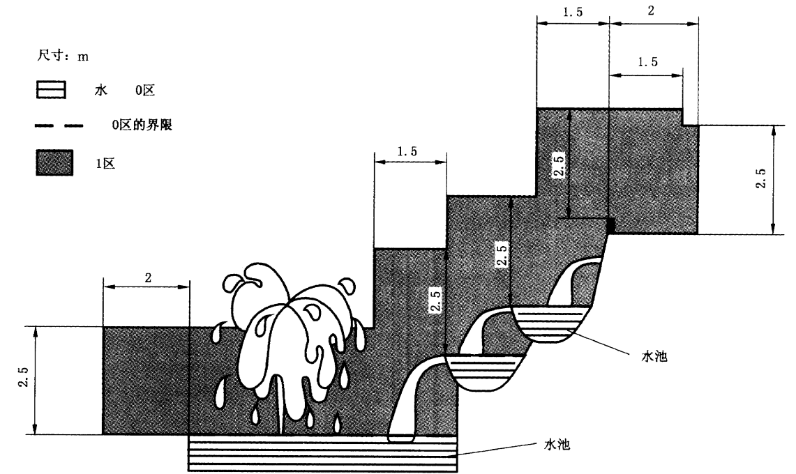
图 702E 确定喷水池的区域示例
