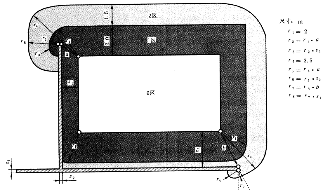
图 702D 装有固定隔板的区域尺寸(平面)示例(装有浴缸的场所另见图 702A)
