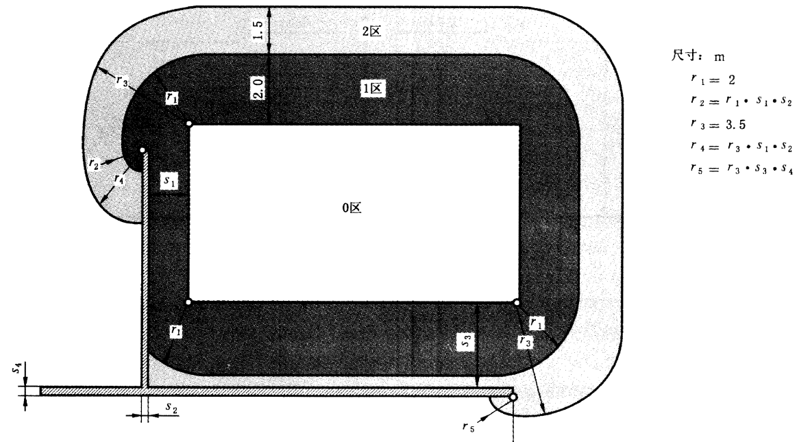
图 702C 装有高度至少为 2.5 m 的固定隔板的区域尺寸(平面)示例
